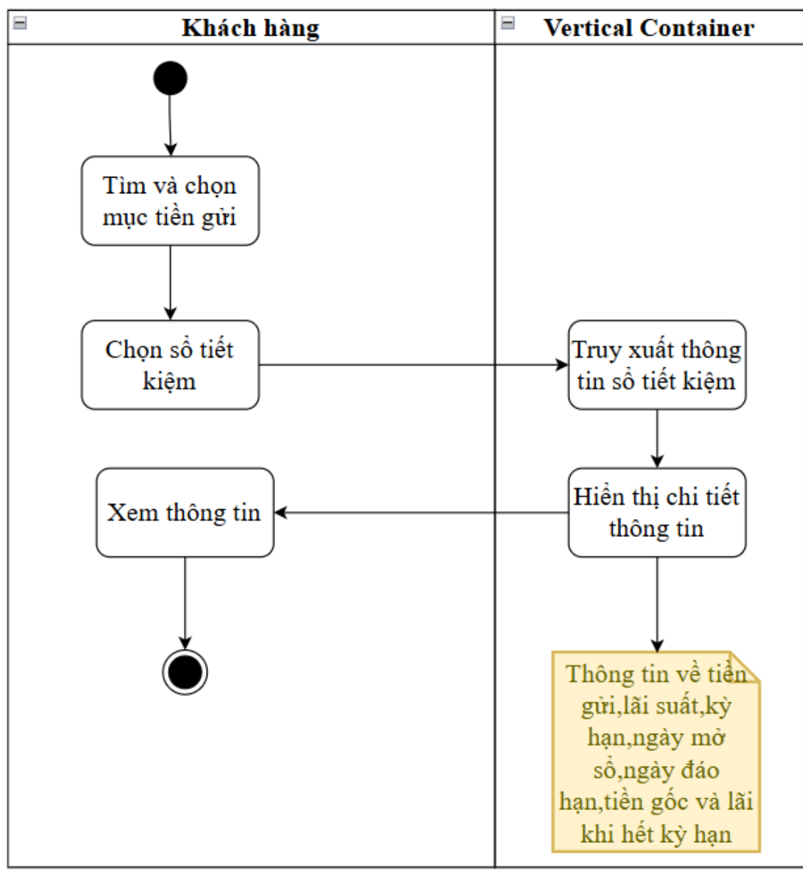
Biểu đồ hoạt động truy vấn thông tin sổ tiết kiệm
