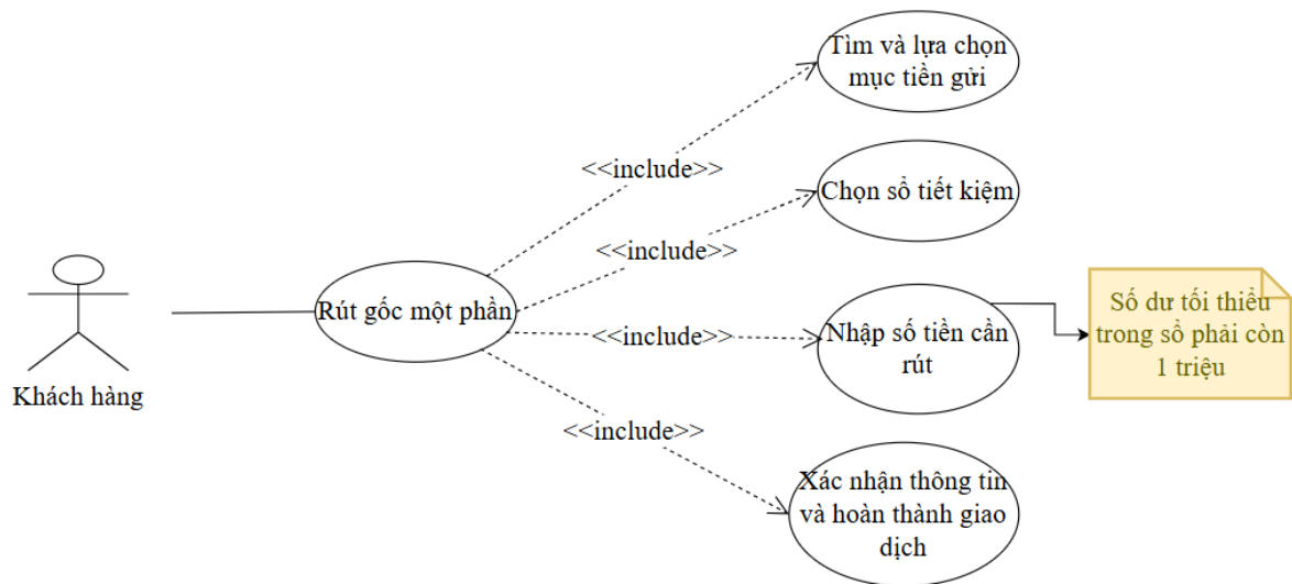
Use Case chức năng rút gốc một phần sổ tiết kiệm
