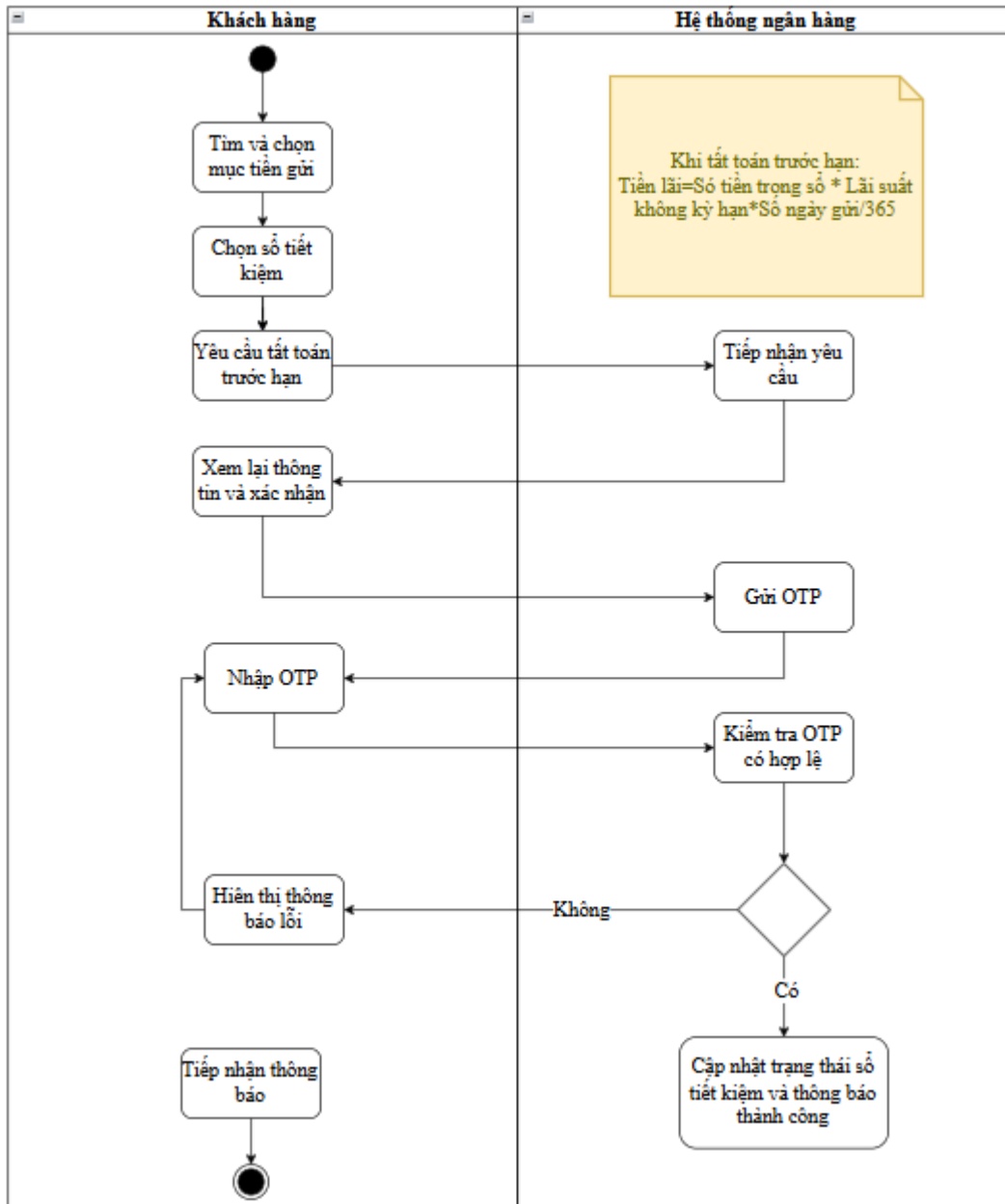
Biểu đồ hoạt động tắt toán trước hạn sổ tiết kiệm
