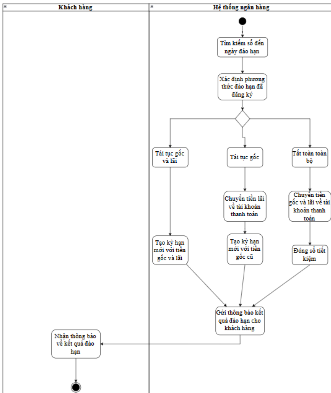
Biểu đồ hoạt động xử lý đáo hạn sổ tiết kiệm
