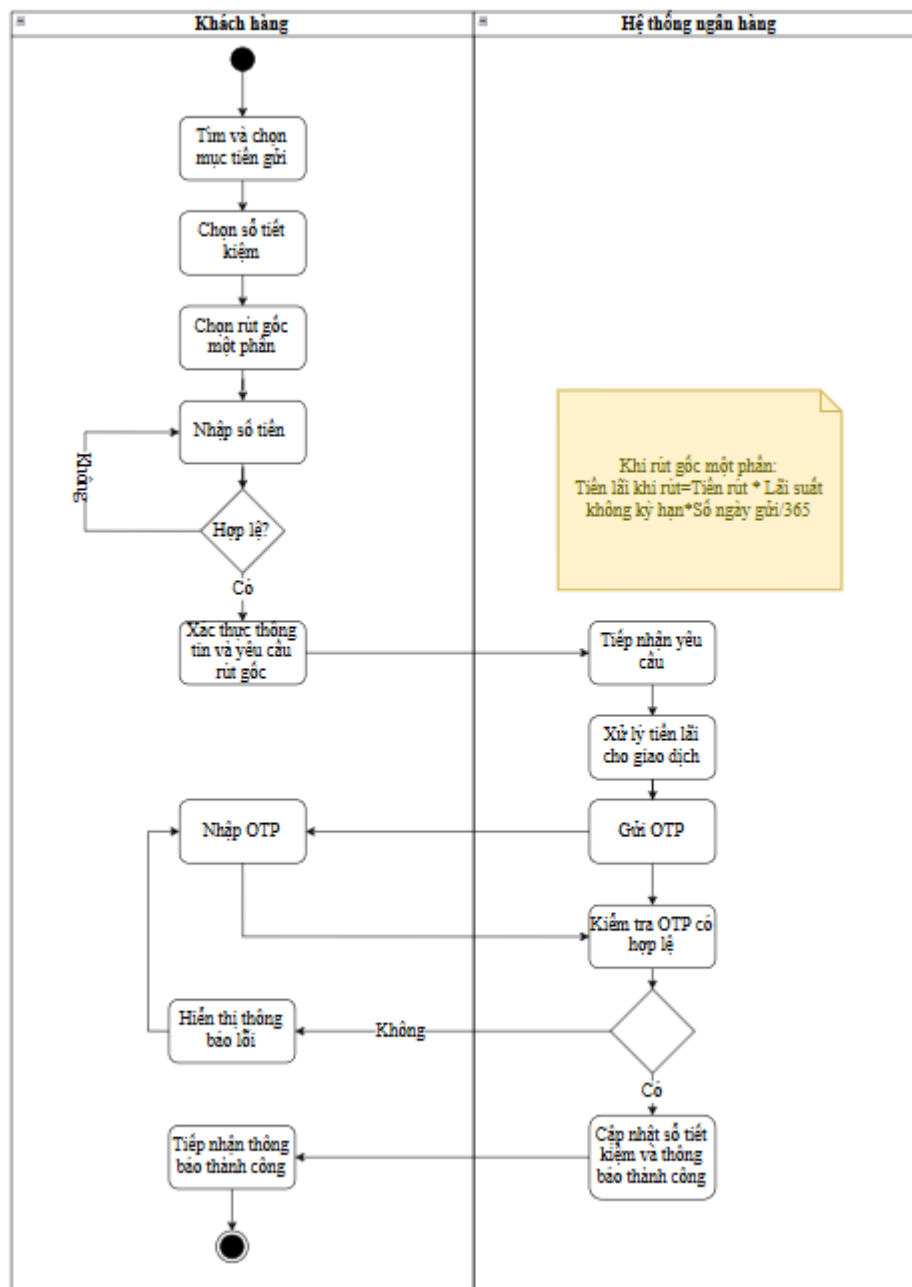
Biểu đồ hoạt động rút gốc một phần số tiết kiệm
