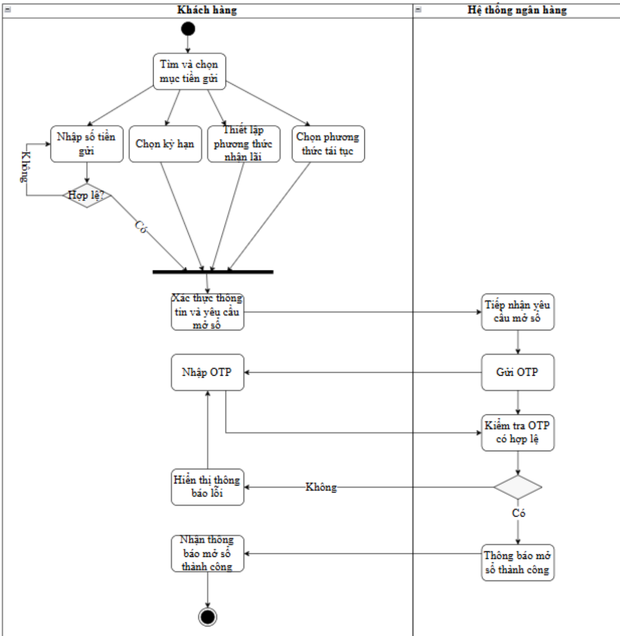
Biểu đồ hoạt động mở số tiết kiệm online
